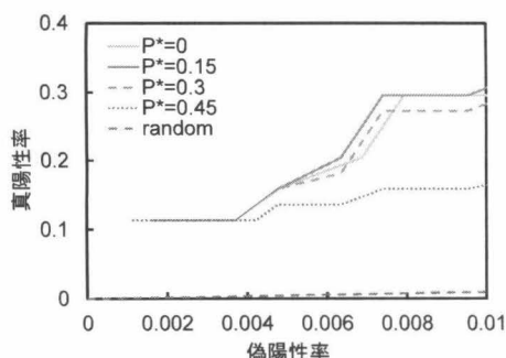
図 6: ROC 0.01 曲線。灰色の破線はランダムな予測における性能を表す。
