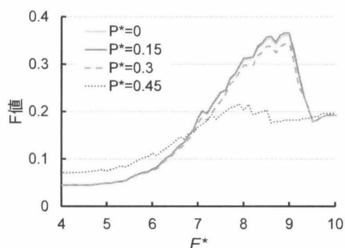
図 5: 提案手法による予測を構造データセットに適用したときの F 値。 P^* = 0 は図 4 と同一の曲線である。
