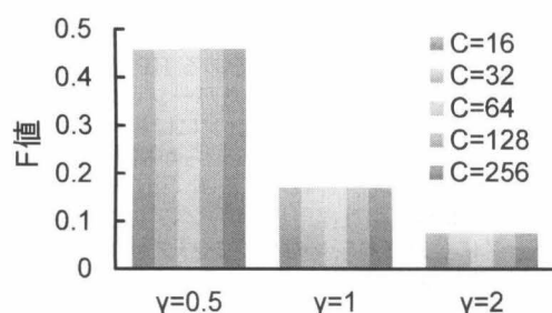
図 3: サポートベクターマシンによる予測を検証用データセットに適用したときの F 値。C と \gamma はサポートベクターマシンのパラメータである。
